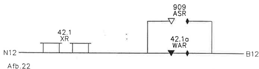
Afb. 22 Aankondiging overweg 42.1
