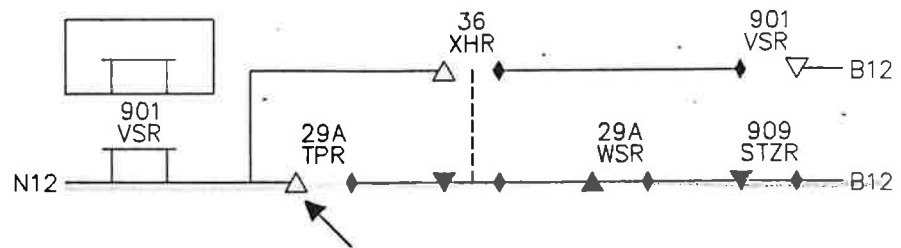
Afb. 16 Rijweg ingesteld
