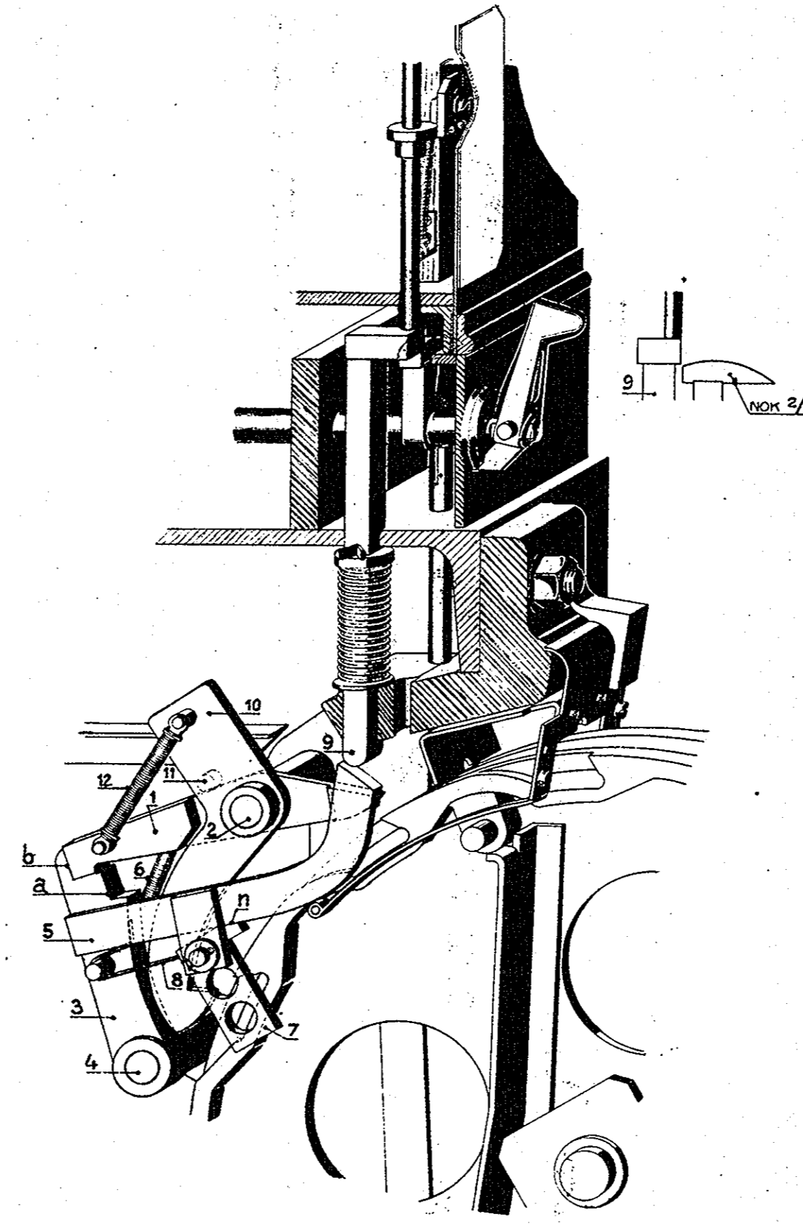
FIG. 1b VENSTER VRIJ KRUKJE NORMAAL
