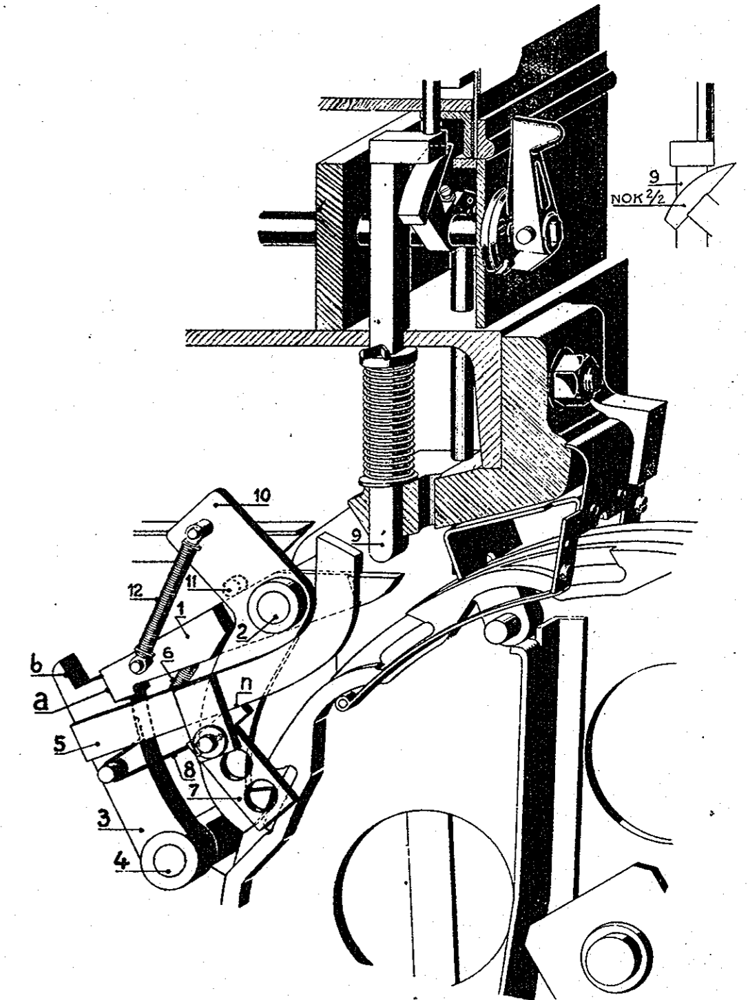
FIG. 1c HANDEL EENMAAL BEDIEND KRUKJE NOG OMGELEGD
